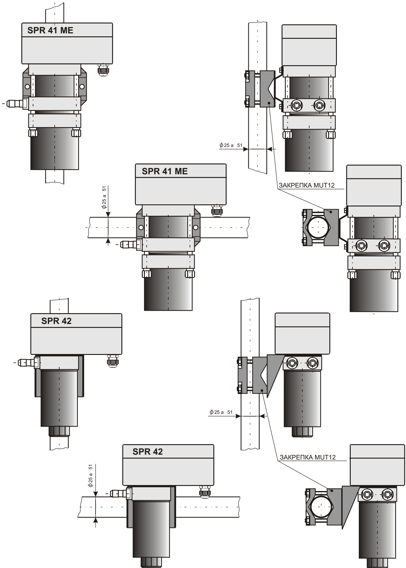
Монтаж датчиков SPR с помощью закрепки MUT 12
