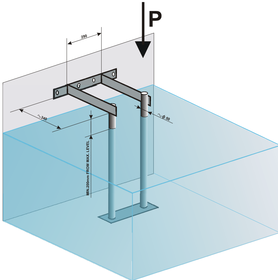
PL 55 Float
