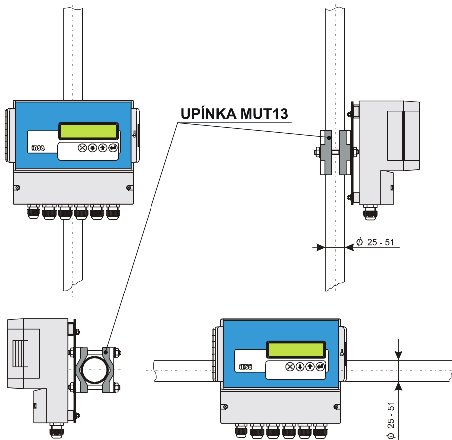
Montáž převodníku řady 66 pomocí upínky MUT 13
