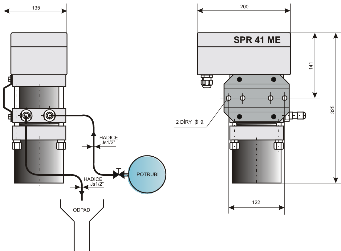
Průtočný snímač SPR 41ME
