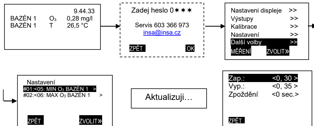
Obr.10. Nastavení mezních hodnot reléových výstupů
