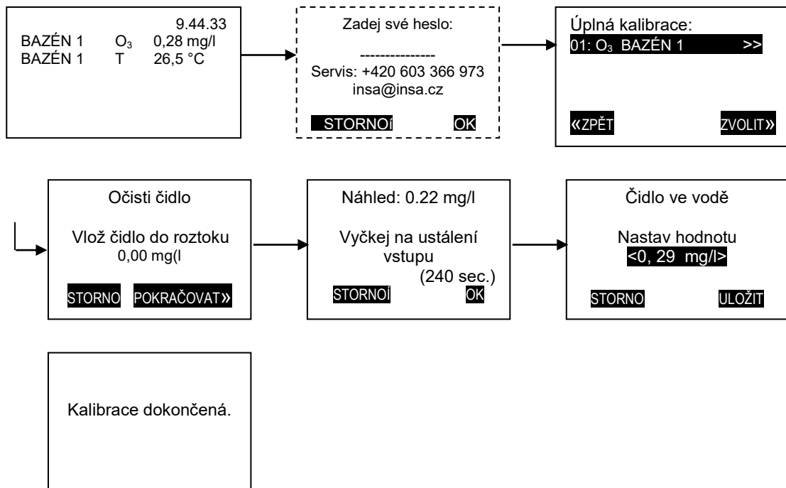
Obr. 7. Dvoubodová kalibrace ozonu
