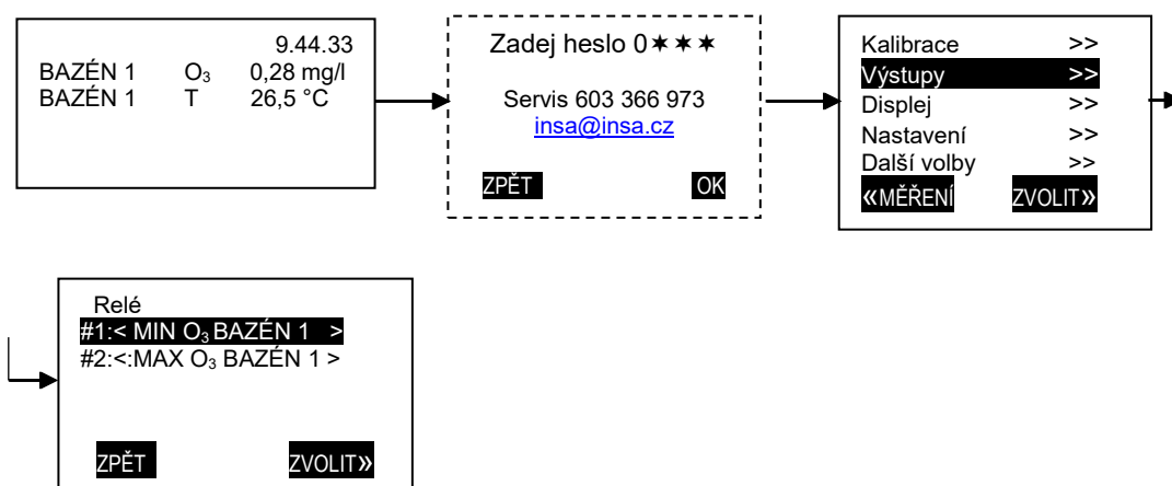
Obr. 9. Nastavení vestavěných reléových výstupů
