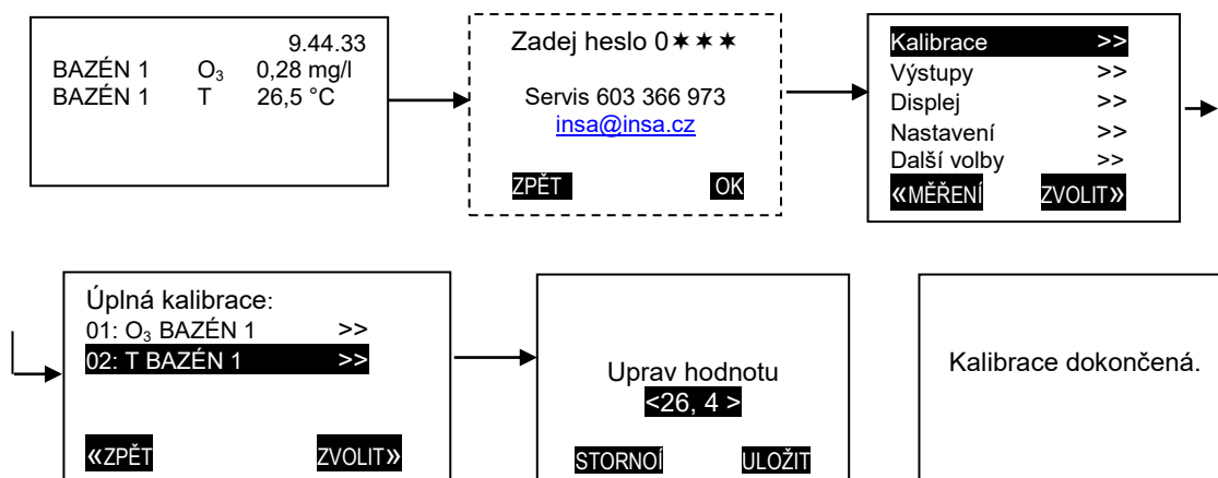
Obr. 8. Kalibrace teplota
