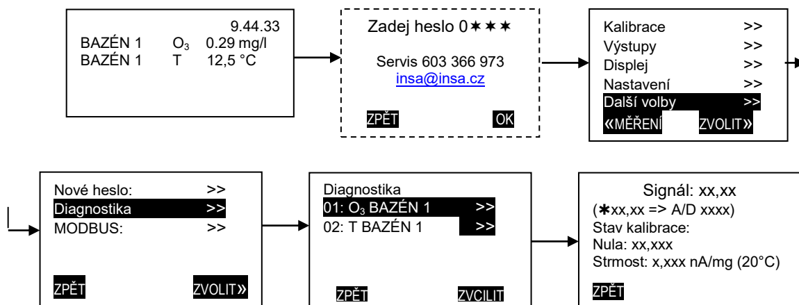
obr.16. Příklad režimu diagnostika – měření ozonu
