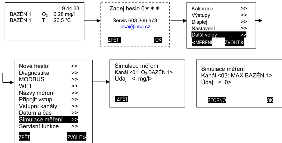
Obr. 14. Simulace měření
