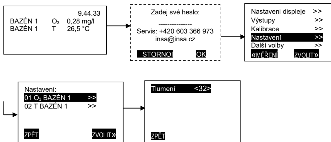
Obr. 13. Zobrazení funkce – tlumení
